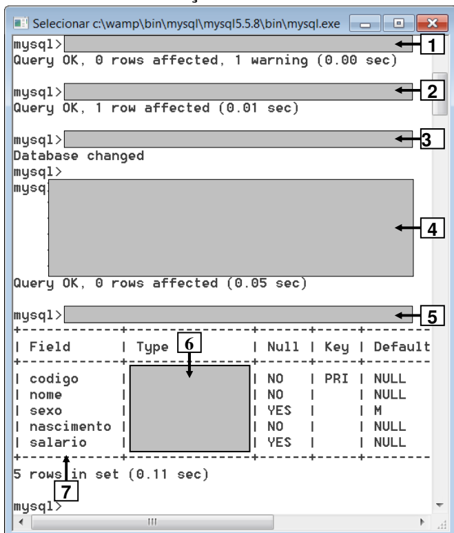
Figura 12(b) - Console do MySQL 5
